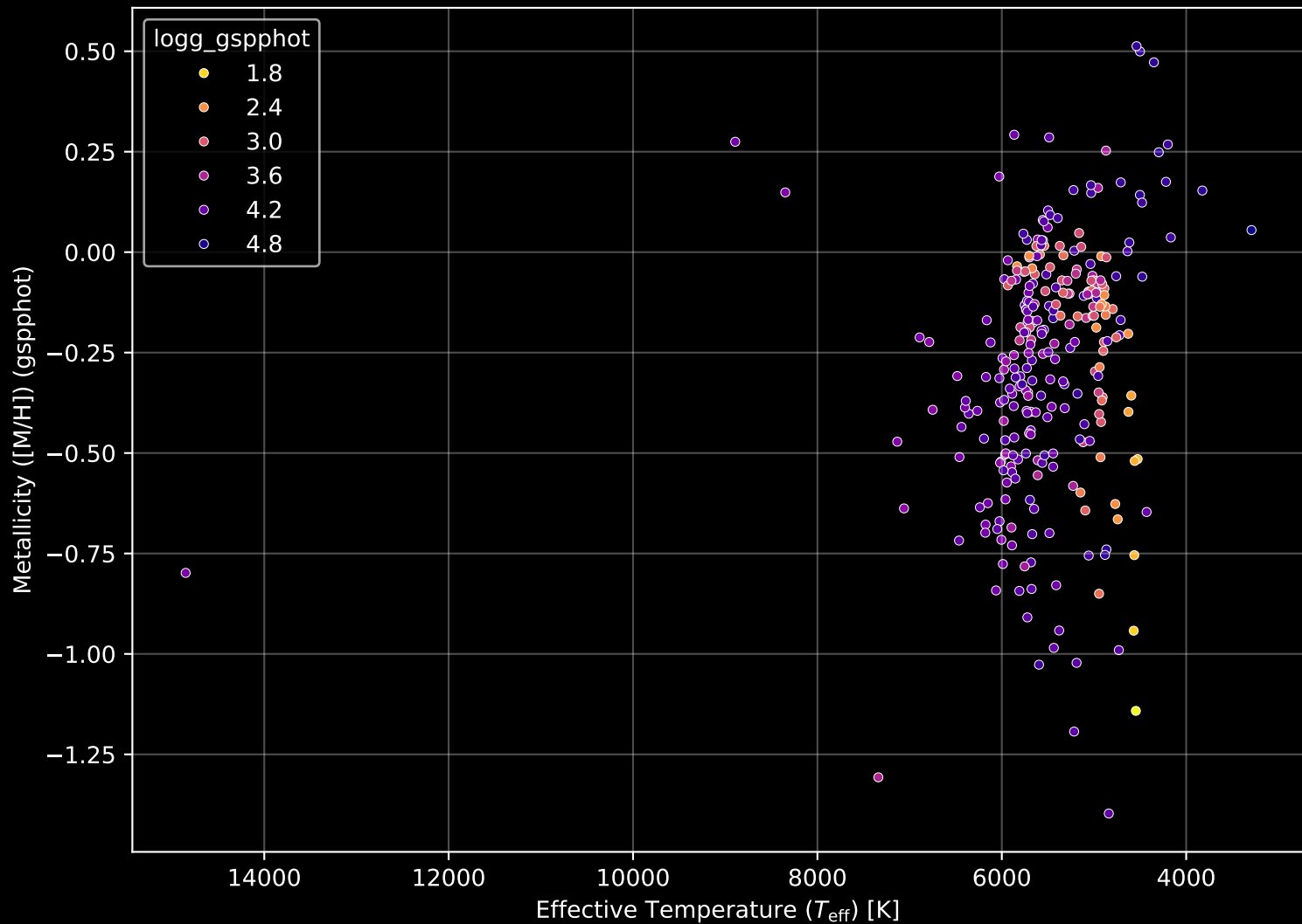
APOGEE DR17 Field: [255-27] Stellar Population Parameters (n= 283)
